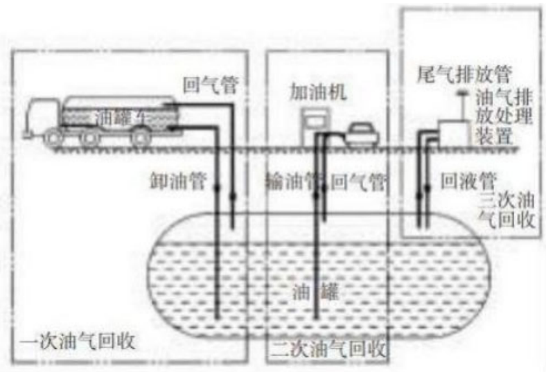
图 4-1 油气回收示意图
