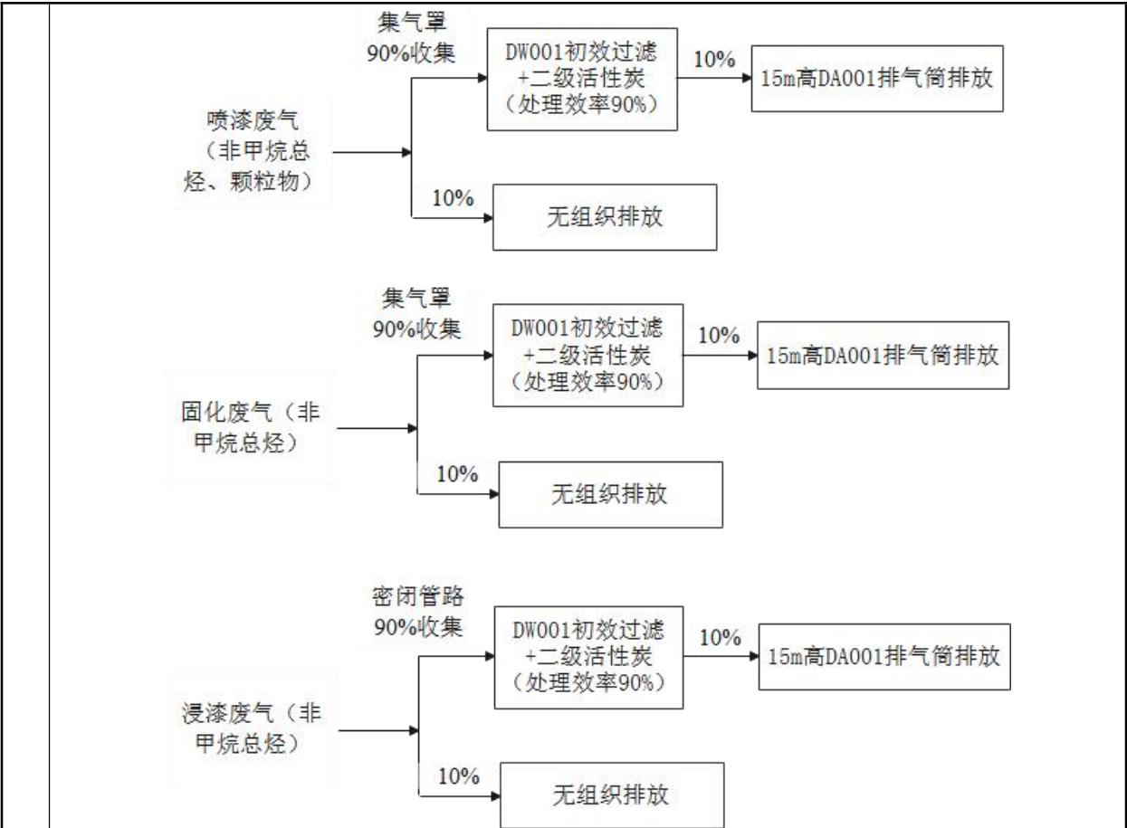
图 4.1-1 本项目废气收集及处理工艺示意图
