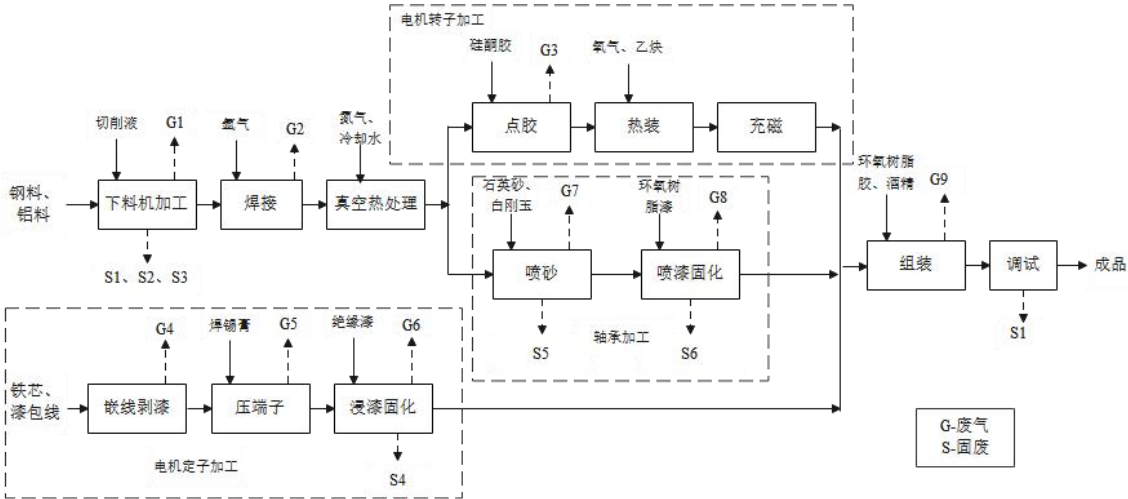
图 2-2 气悬浮高速旋转流体机械设备工艺流程和产污环节图
